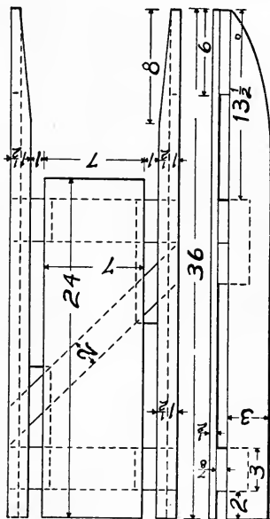
Fig. 337—Sled
